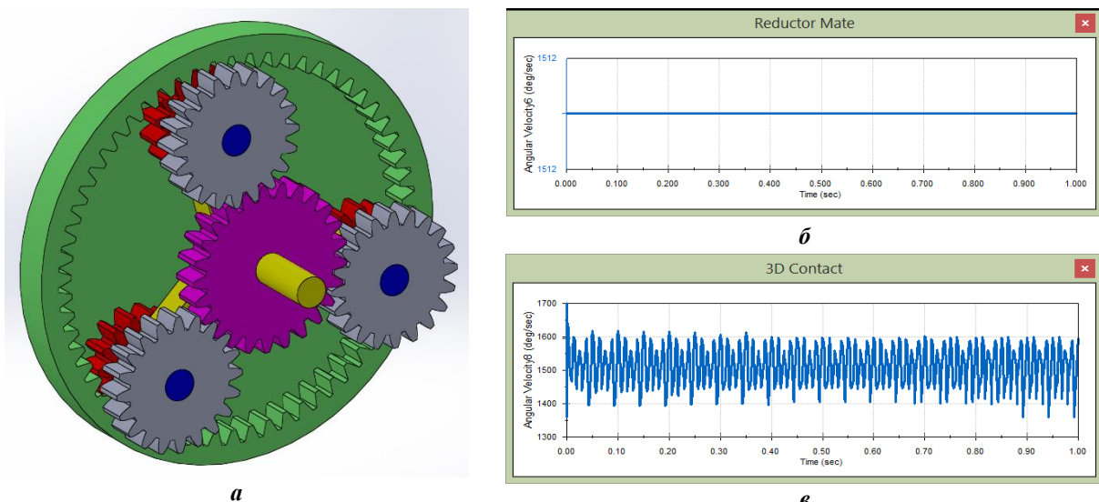
Рис. 8. Моделювання планетарної передачі: а – 3D-модель; б – кутова швидкість вихідної ланки, отримана при використанні функції «Редуктор»; в – кутова швидкість вихідної ланки, отримана при використанні функції «3D-контакт»
