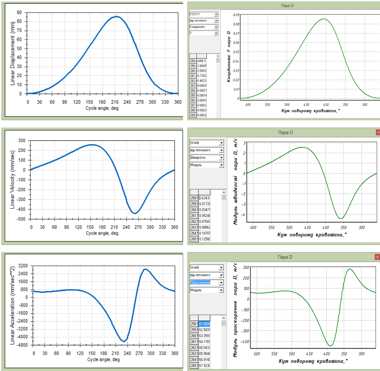
Рис. 3. Закони руху вихідної ланки важільного механізму: а – отримані за допомогою SOLIDWORKS Motion; б – отримані за допомогою аналітичних методів
