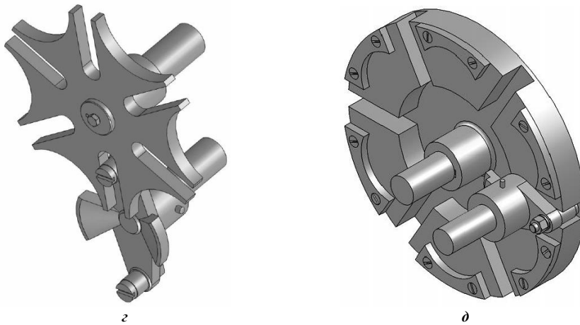
Рис. 1. SOLIDWORKS-моделі мальтійських механізмів
