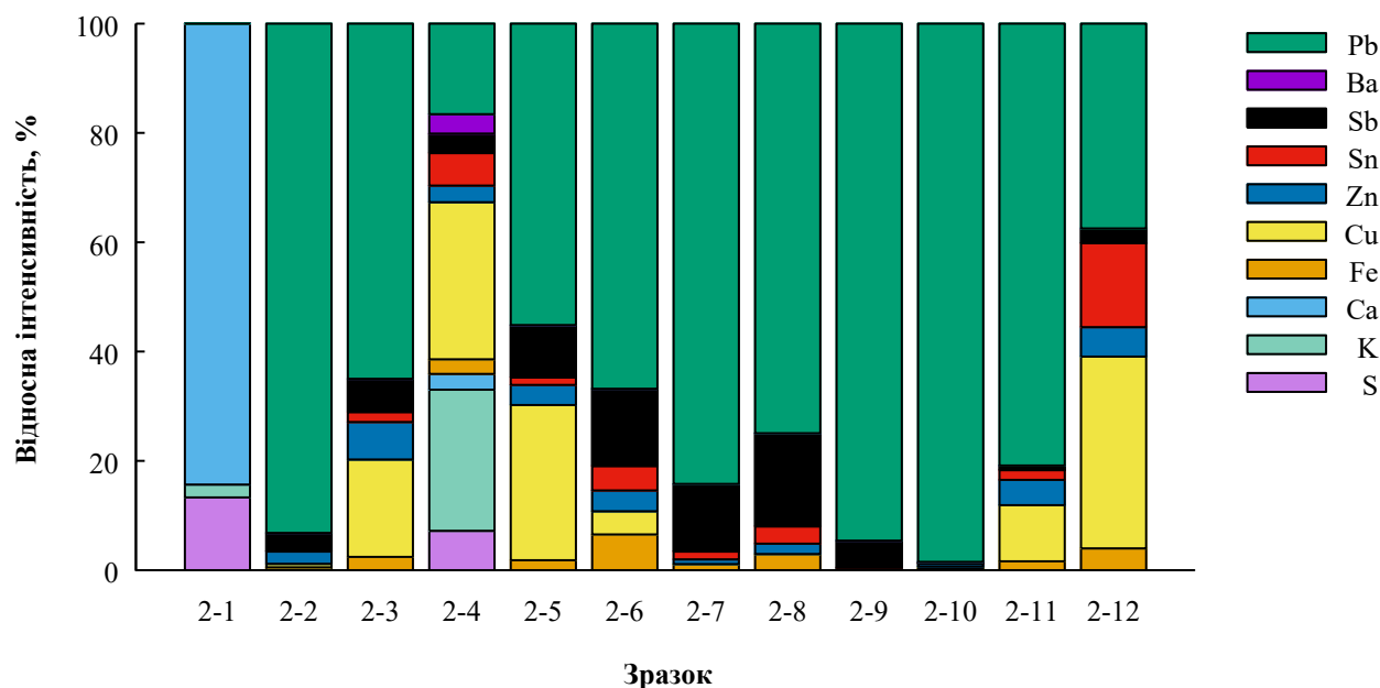
Рис. 2. Стегова діаграма відносні інтенсивностей у відсотках К- та L-серій елементів у зразках продуктів пострілу
