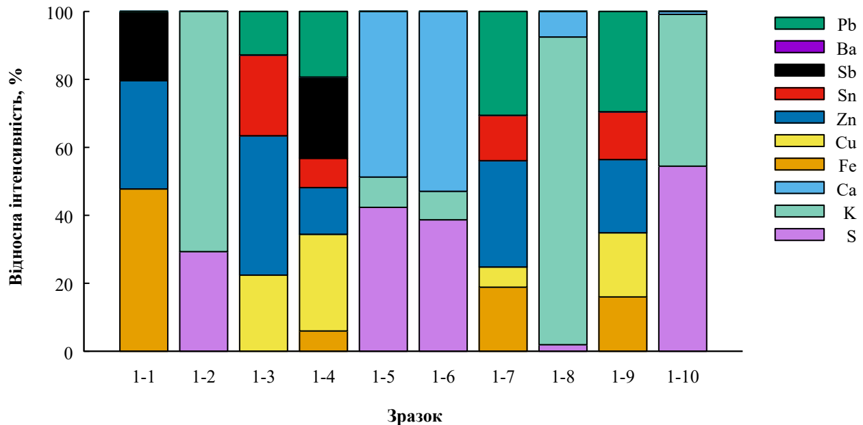
Рис. 1. Стекова діаграма відносних інтенсивностей у відсотках К- та L-серій елементів у зразках порошу
